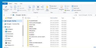
Storegate Sync
