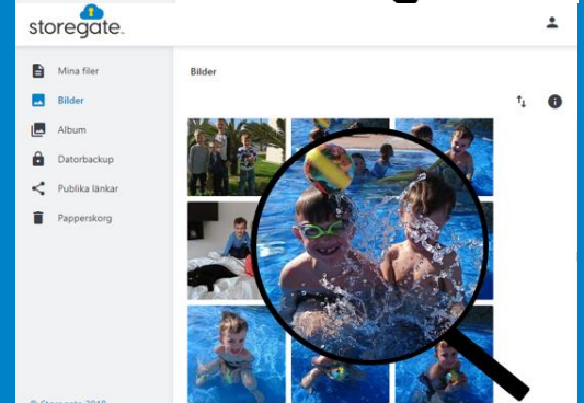
Storegate Webbtjänst
