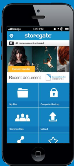
Mobila appar
